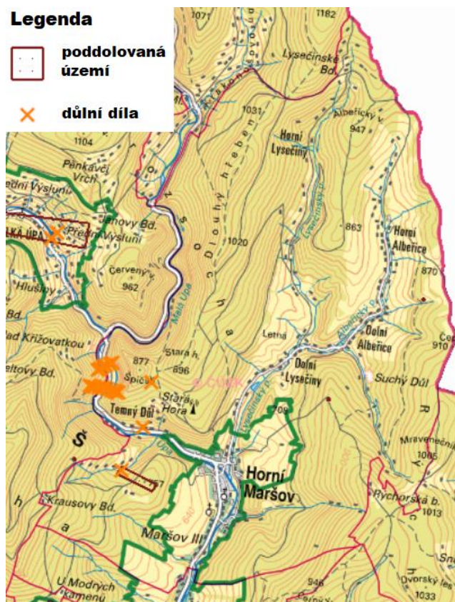
Obrázek 4: Poddolované plochy zasahující do území obce Horní Maršov a důlní díla na území obce Horní Maršov
