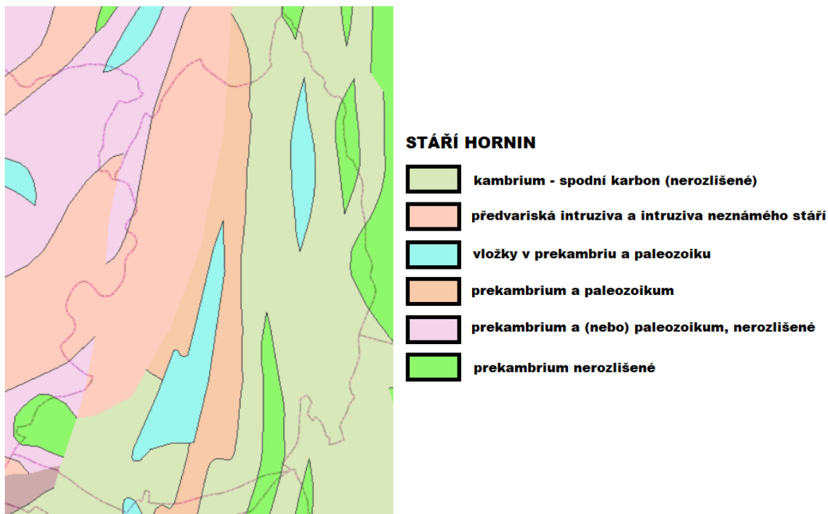
Obrázek 3: Geologické složení území obce Horní Maršov
